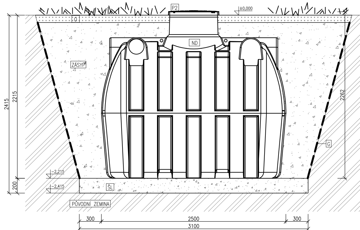
ŘEZ osazení ve volném terénu
