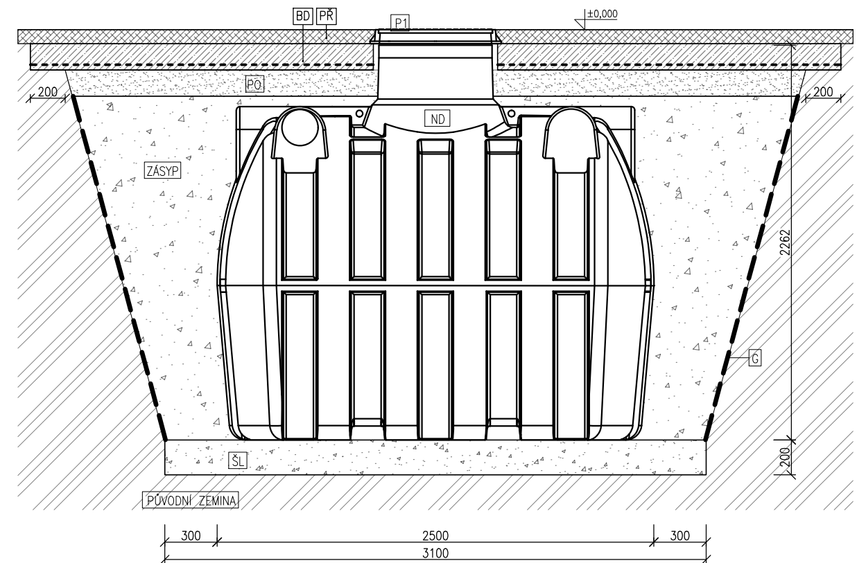
ŘEZ osazení pro pojezd
